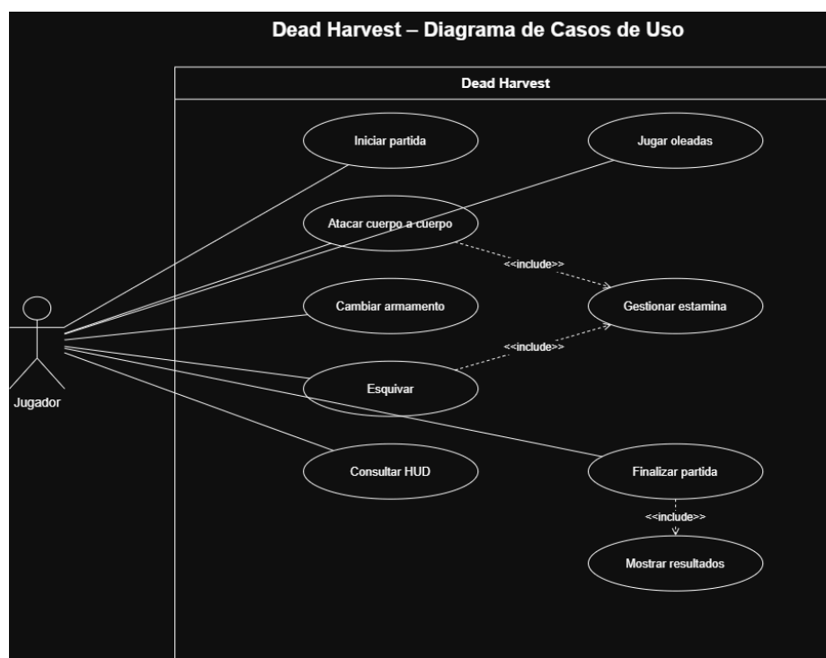
Figura 1. Diagrama de casos de uso — Dead Harvest.
