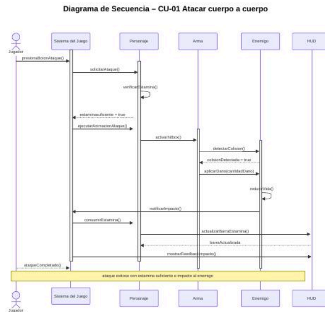
Figura 4. Diagrama de secuencia — flujo principal de ataque exitoso.
