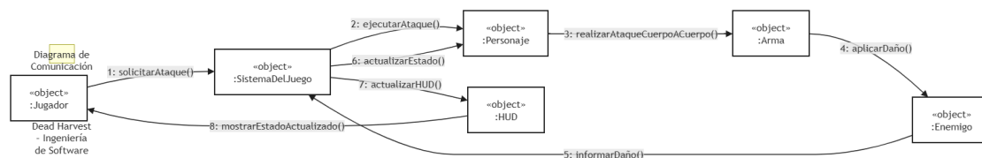
Figura 3. Diagrama de comunicación — CU-01 Atacar cuerpo a cuerpo.
