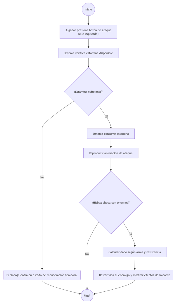
Figura 2. Diagrama de actividades — CU-01 Atacar cuerpo a cuerpo.
